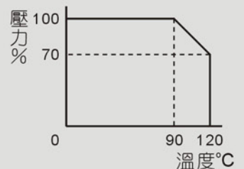
EPDM之壓力溫度特性
