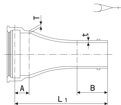
■ 承插式縮管
