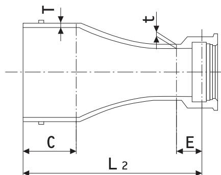
■ 插承式縮管
