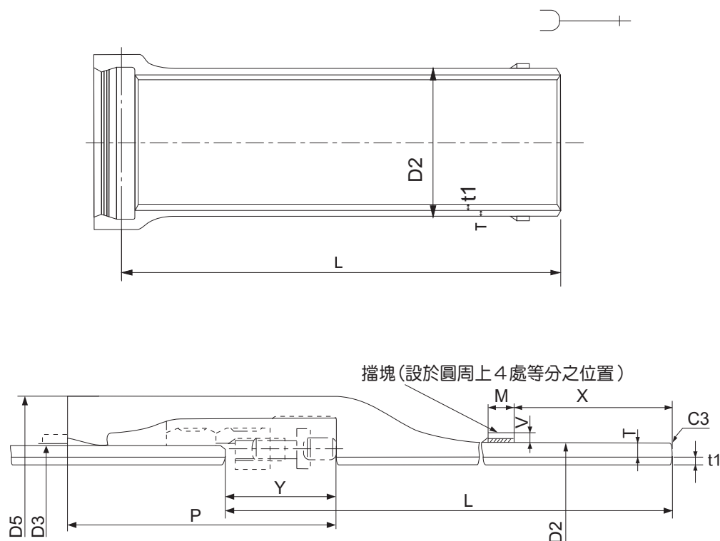
■ 接合部詳細
