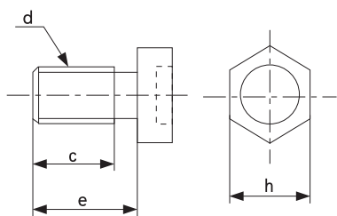
■ 螺 栓
