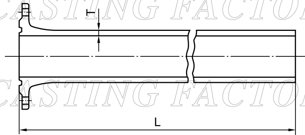
■ 單凸緣長管
