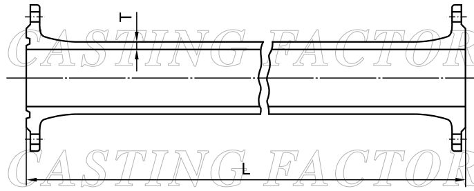
■ 雙凸緣長管
