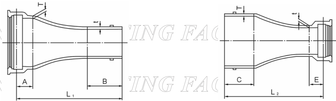
■ 承插式縮管
