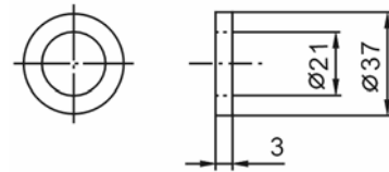
■中間圈用卡具用墊圈 ( CNS 3270-304 )
