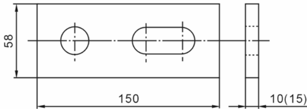
■中間圈用卡具 ( CNS 2473-SS 400 或尼龍 6 )
