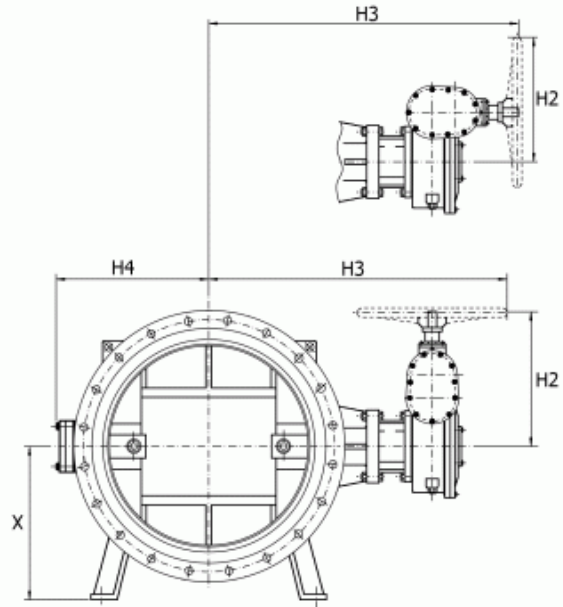
■ 長體型蝶閥-單閥瓣臥式 Long Body Type Butterfly Valves (Single Disc & Horizontal Type)
