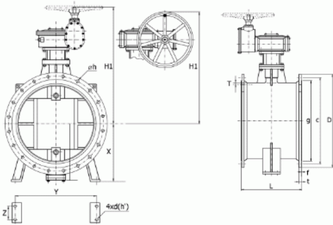
■ 長體型蝶閥-單閥瓣立式 Long Body Type Butterfly Valves (Single Disc & Vertical Type)
